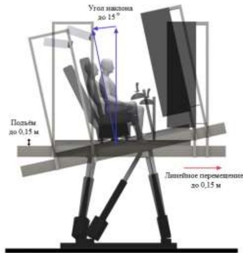
Рисунок 3 - Требуемые движения системы подвижности тренажёра
