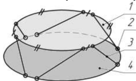
1 – подвижная платформа; 2 – шарнирное соединение; 3 – пневмоцилиндр; 4- неподвижное основание.
