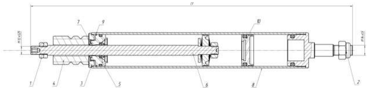
Рис. 2. Схема однотрубного амортизатора передней подвески
