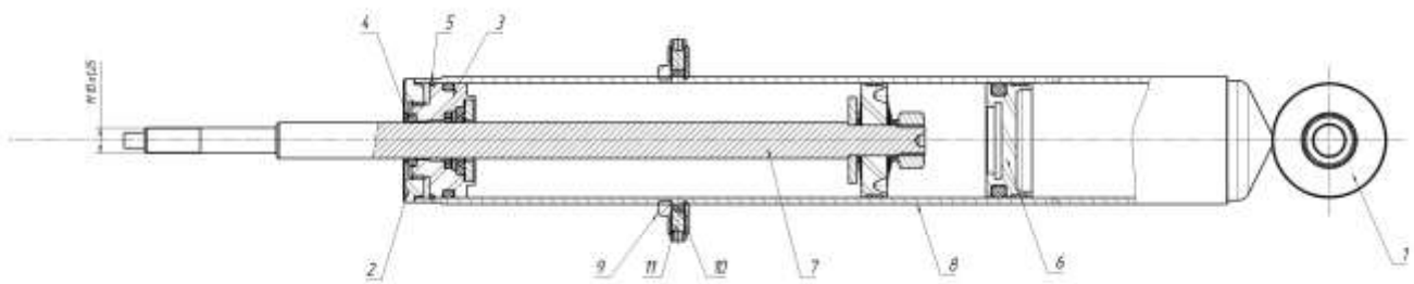
Рис. 1. Схема однотрубного амортизатора задней подвески
