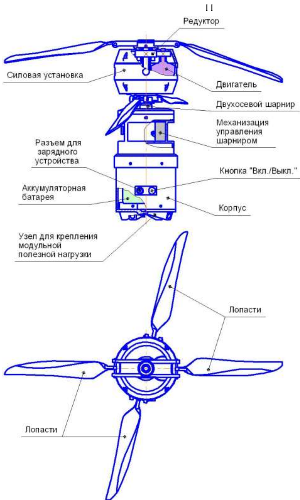
Рисунок 1 – Конструкция ДПЛА «Оса».
