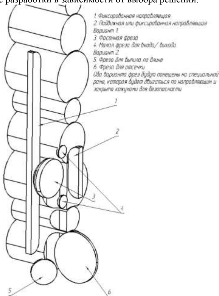
Рис. 2. Схема комплекса.
