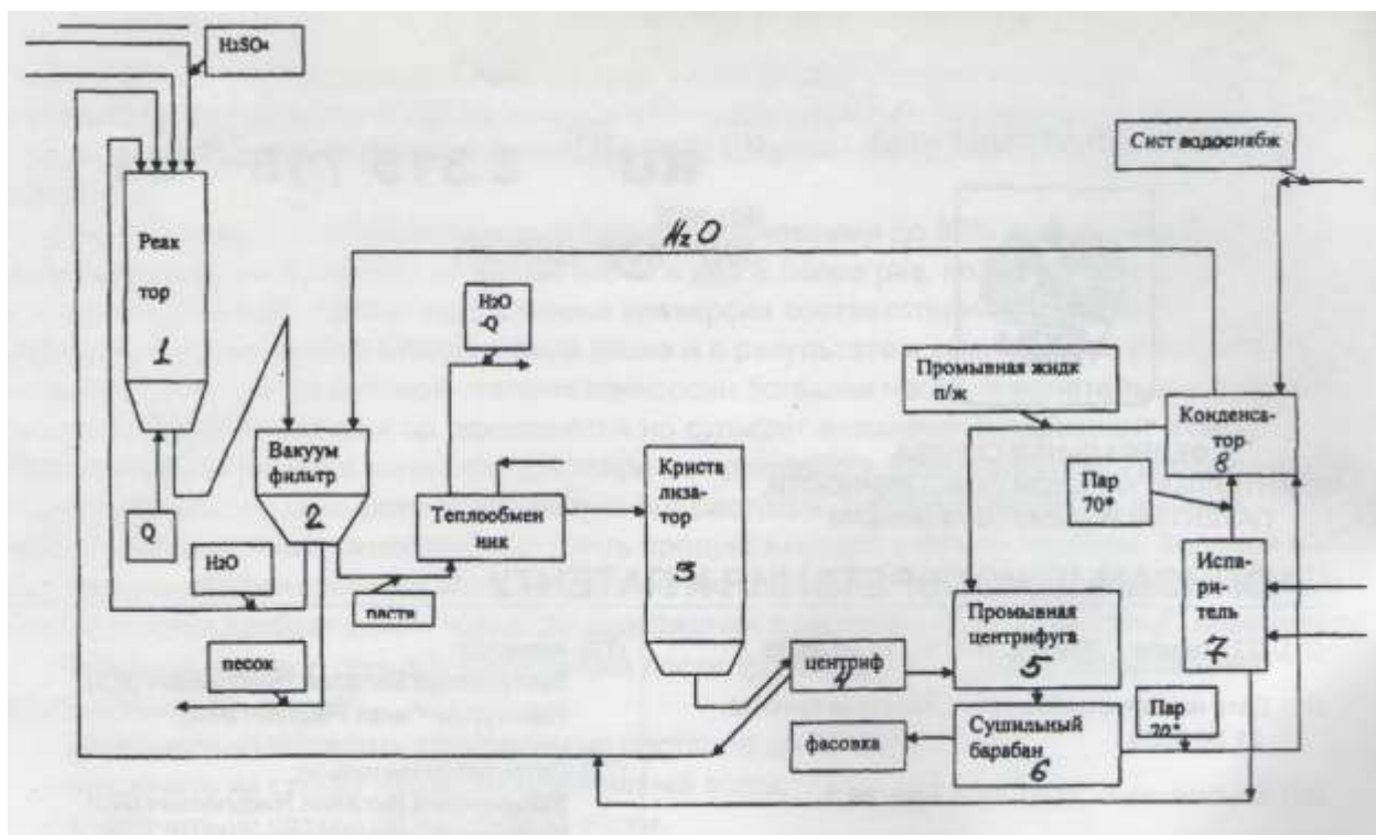
Рис.1. - Структурная схема получения сульфата алюминия.
