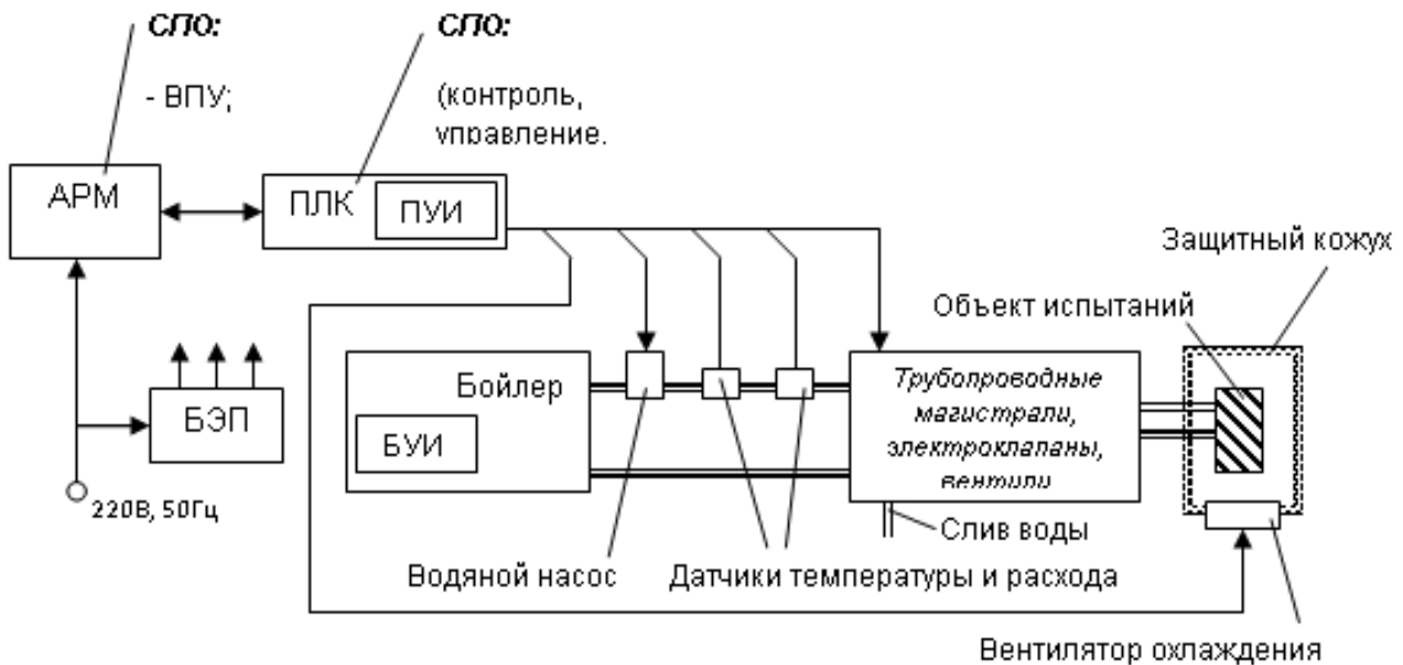
Рис. 2 Структура АСИ-РОМ.
