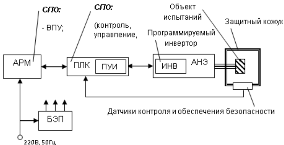
Рис.1 Структура АСИ-КСО.
