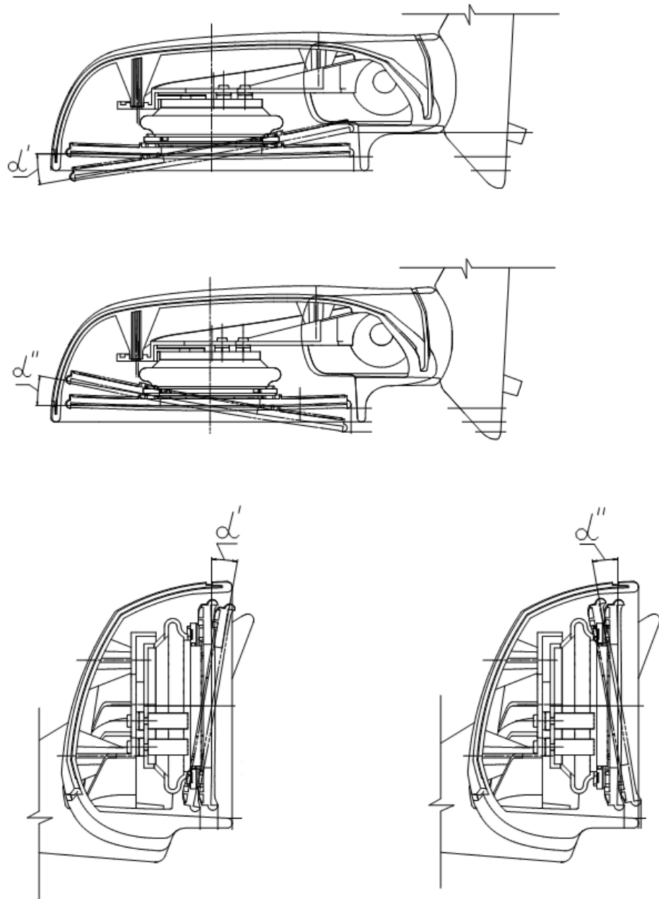
Рис. 1 Углы регулировки бокового зеркала заднего вида
