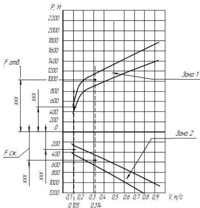
Рис. 1. Скоростная характеристика стоек
