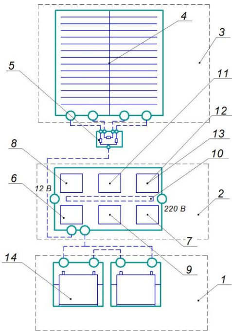
Рисунок 1 – Блок схема комплекса
