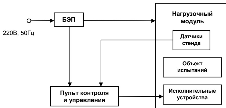
Рисунок 4 – Структура технических средств стенда
