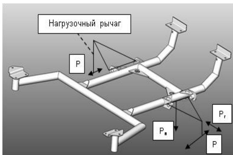
Рисунок 2 – Схема приложения сил при проведении прочностных статических испытаний
