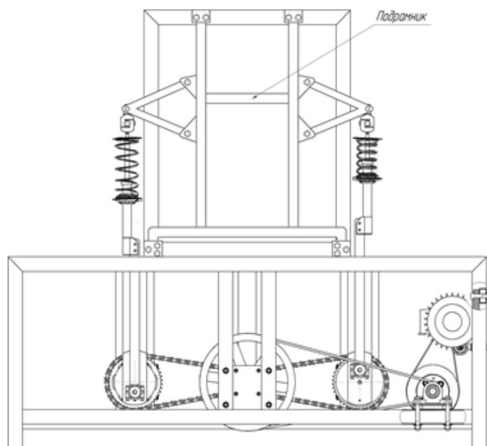
Рисунок 1 – Вариант схемы фрагмента нагрузочного модуля испытательного стенда
