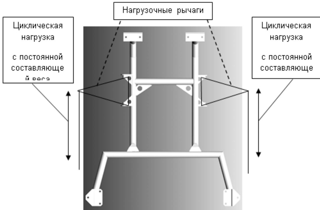
Рисунок 3 – Схема приложения сил при проведении ресурсных испытаний подрамника на усталостную прочность
