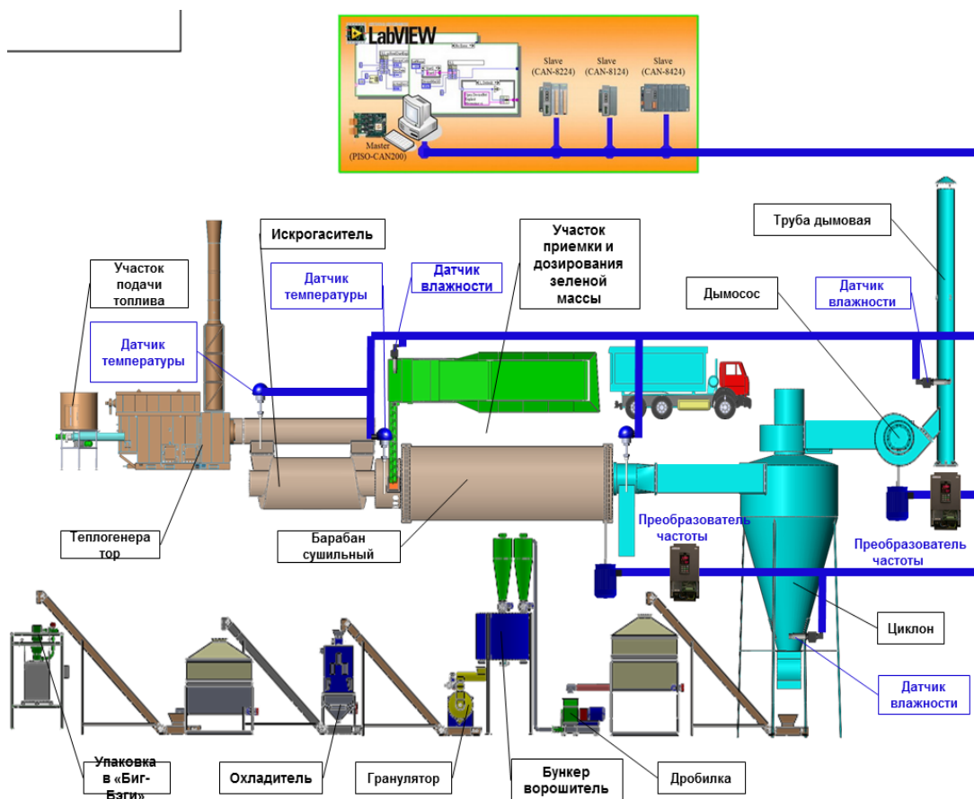
Рис.1. Схема существующей линии по производству ВТГ с расположением модернизируемых элементов
