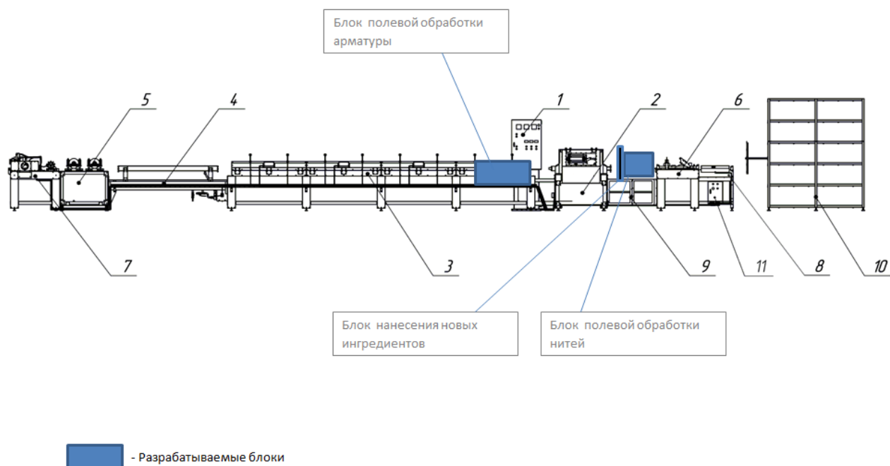
Рис. 1 Существующая линия по производству полимерной арматуры А-001-2013ТП со встроенными узлами установки. 1. Блок питания и управления. 2. Узел обмотки нити. 3. Печи полимеризации. 4. Блок охлаждения нити. 5. Протяжной блок нити. 6. Пропиточная ванна. 7. Отрезное устройство. 8. Блок снятия замасливателя с нити. 9. Блок полевой обработки нити+ блок нанесение новых ингредиентов. 10. Шпулярник. 11. Натяжитель нити.
