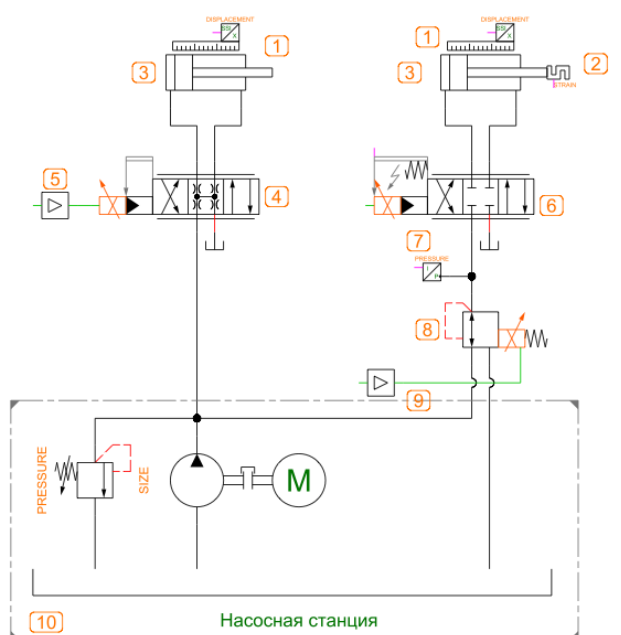
Рисунок 1 - Принципиальная гидравлическая схема
