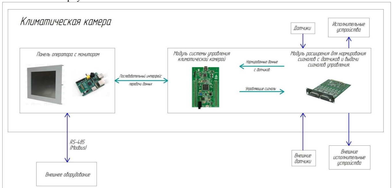
Рис. 1. Принципиальная схема системы
