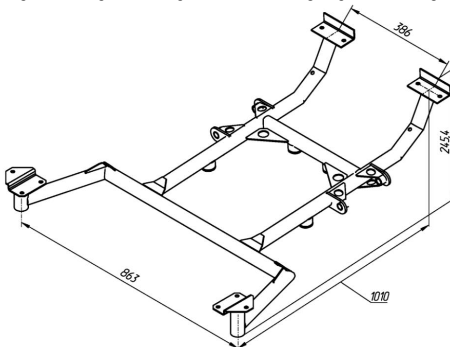
Рис.2. Базовый вариант подрамника
