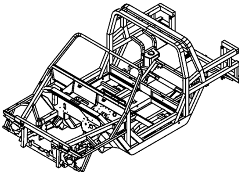
Рис.1. Пространственная рама легкого внедорожного транспортного средства с усилителями в зонах соединения узлов каркаса
