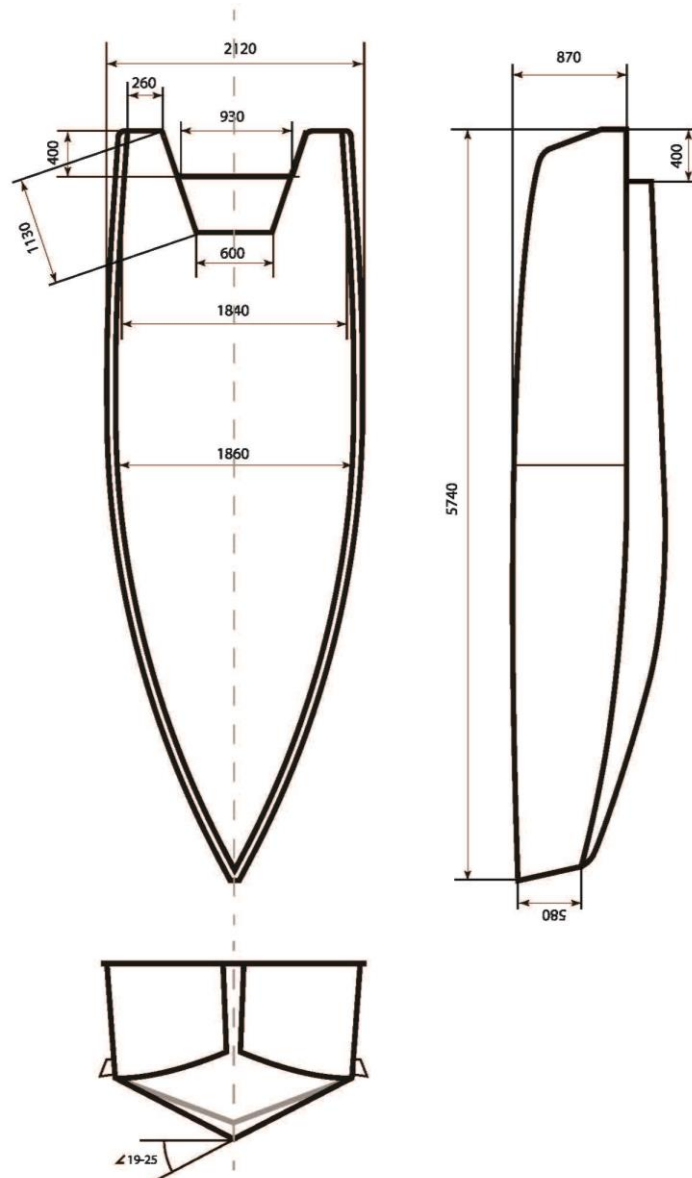
Рис.1 Базовые габаритные размеры
