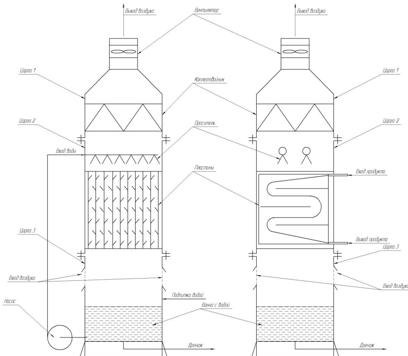
Рис.1. Принципиальная схема АВВО
